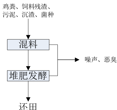
图 3.3-3 堆肥发酵工艺流程图
