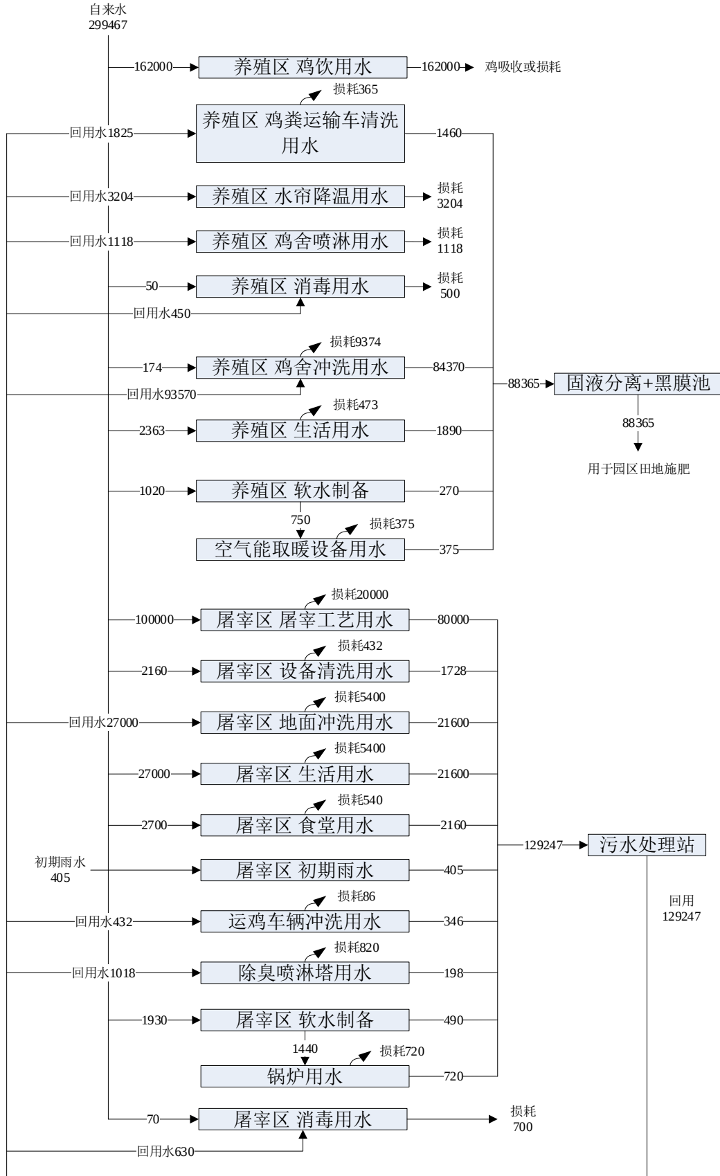
图 3.5-1 全厂项目近期（2025 年~2027 年）水平衡图（单位：m³/a）
