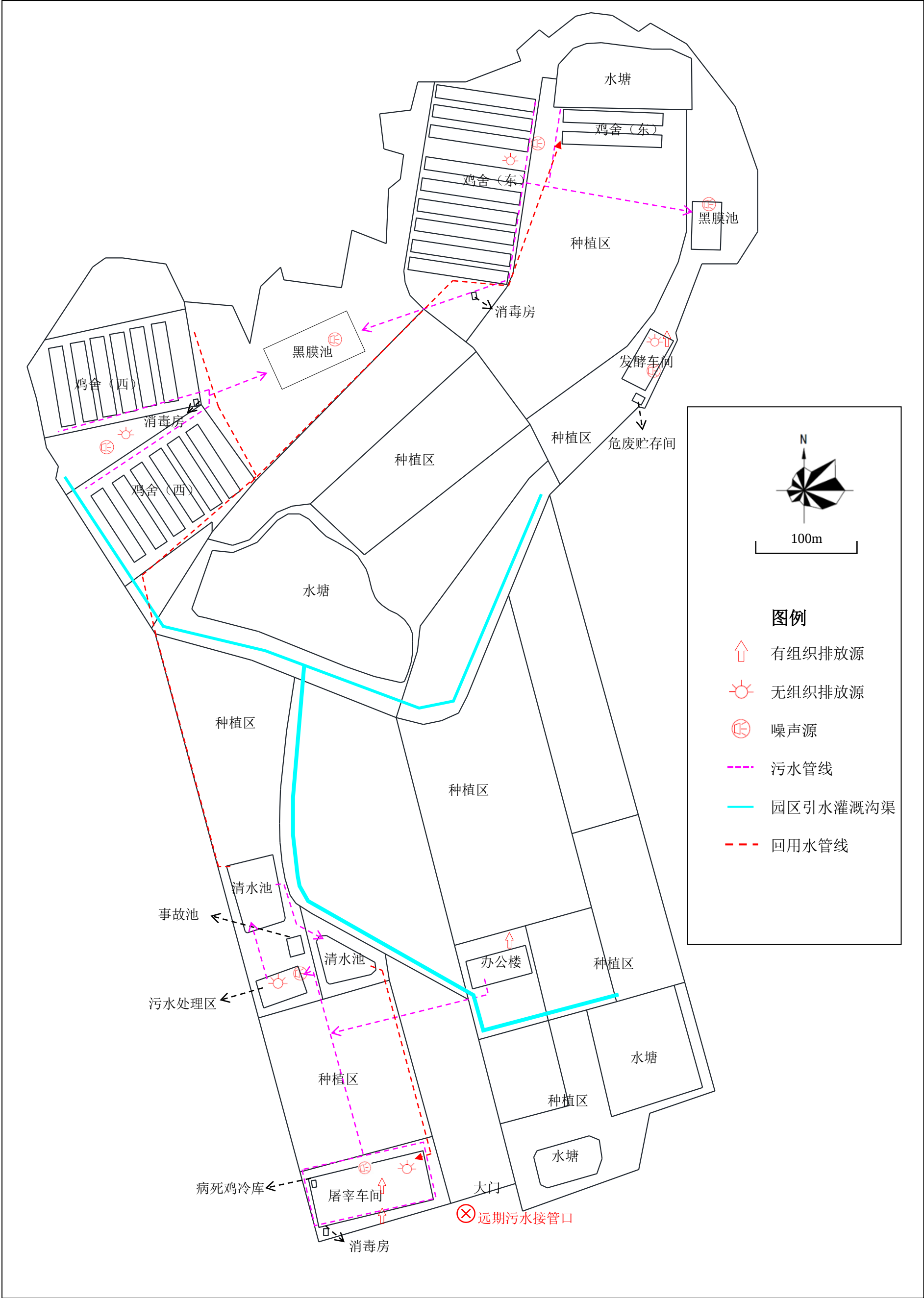
图 3.2-2 本项目建成后全厂平面布置图
