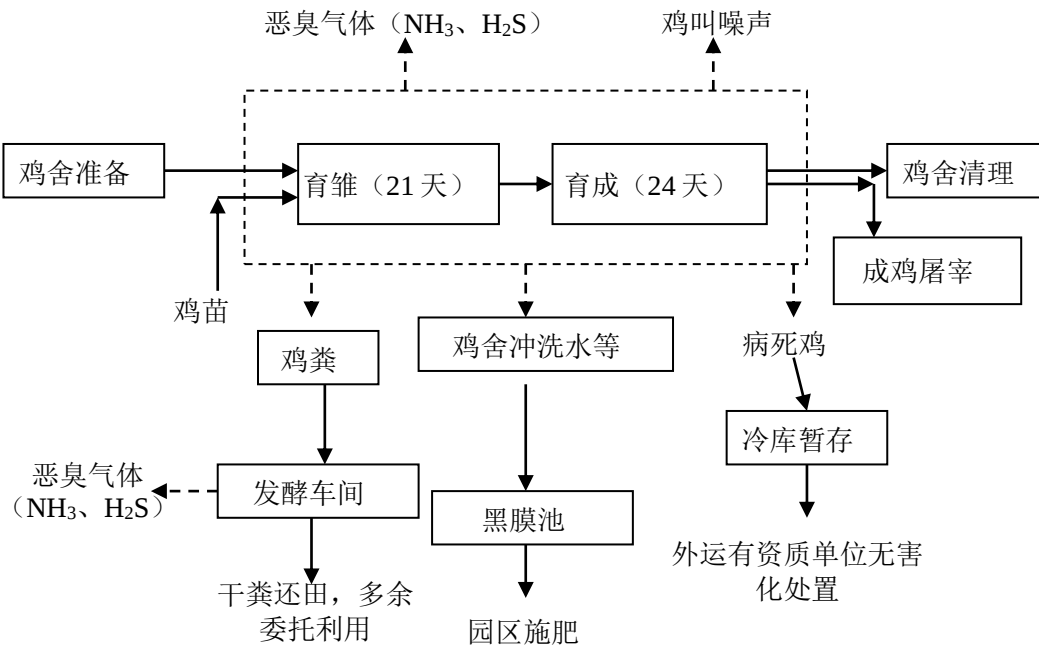
图 3.3-1 养殖工艺流程图
