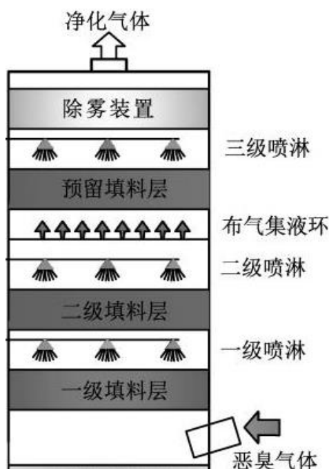
图 6.2-2 本项目生物喷淋塔原理图
