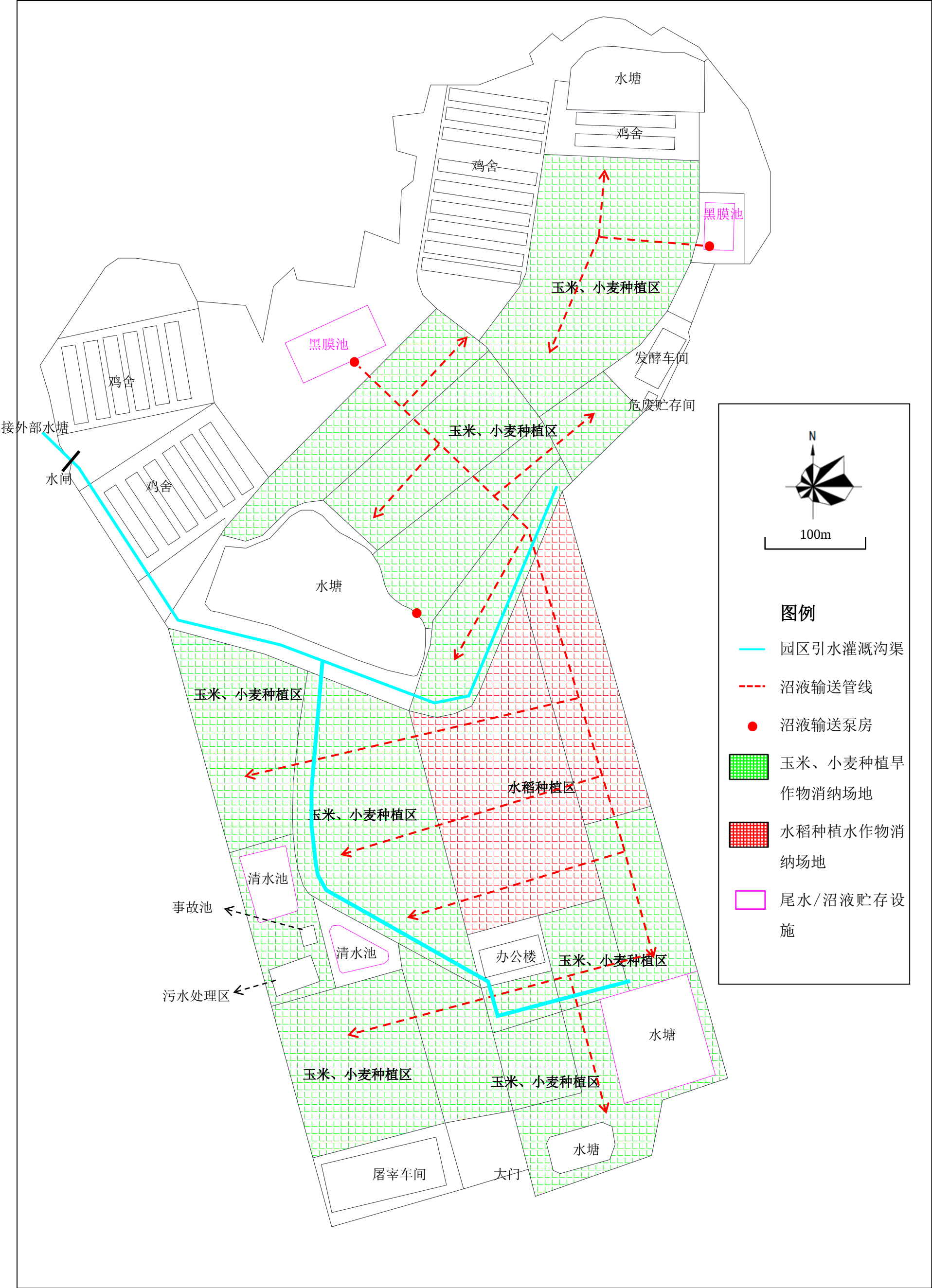
图 3.3-4 本项目沼液输送系统、消纳场地等分布图
