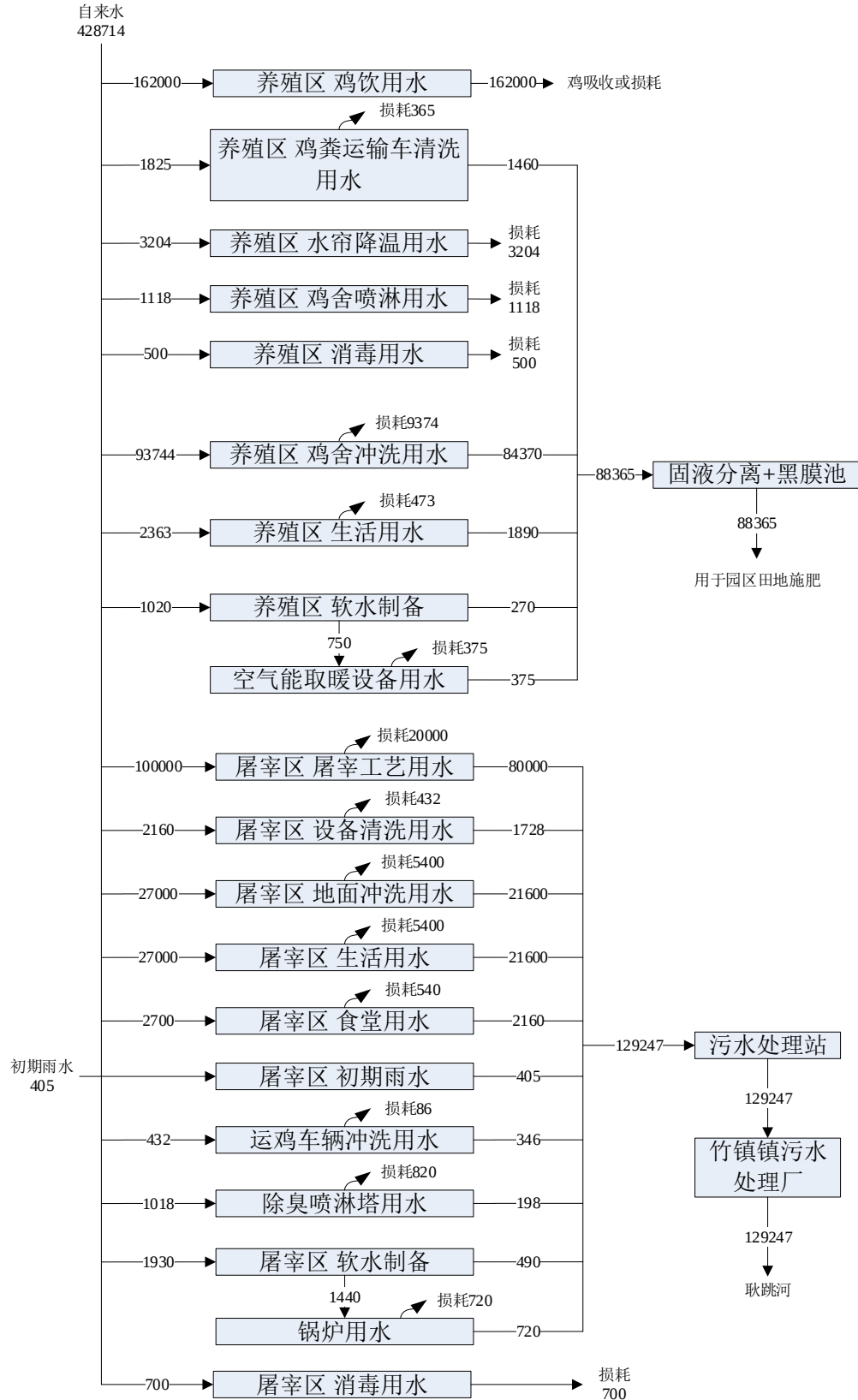
图 3.5-2 全厂项目远期（2028 年起）水平衡图（单位：m³/a）
