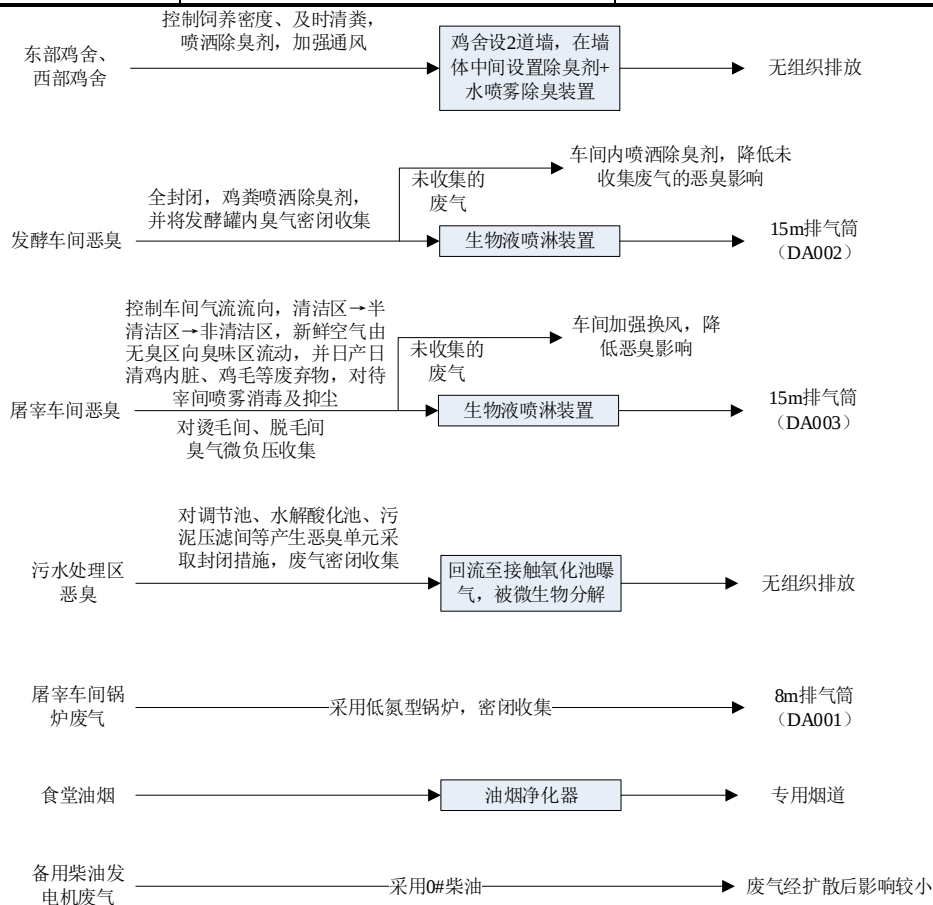
图 6.2-1 废气污染防治流程图
