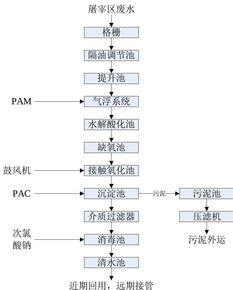
图 6.2-4 污水处理工艺流程
