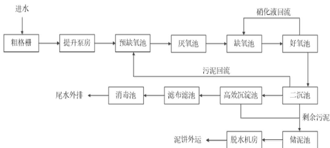
图 5.2-8 六合区竹镇镇污水处理厂处理工艺流程图
