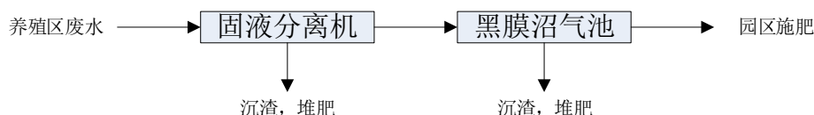
图 6.2-3 污水处理工艺流程
