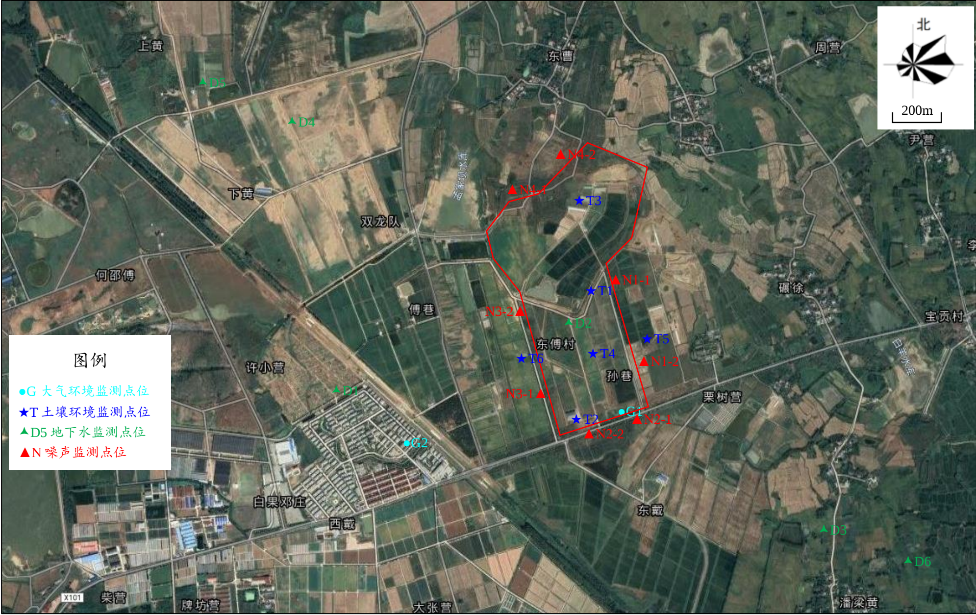
图 4.2-1 大气、土壤、地下水及噪声监测点位图
