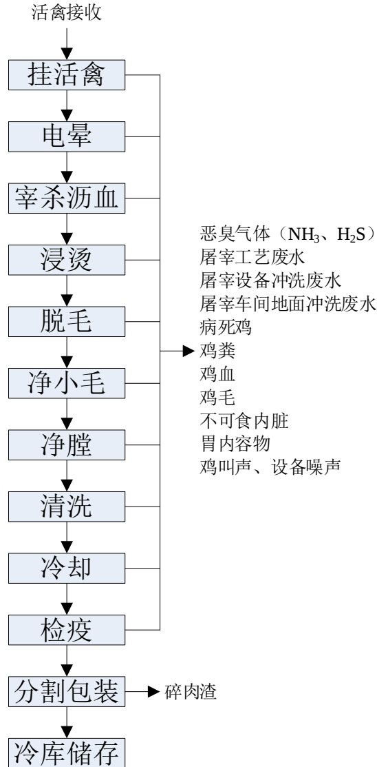
图 3.3-2 肉鸡屠宰工艺流程及产污环节
