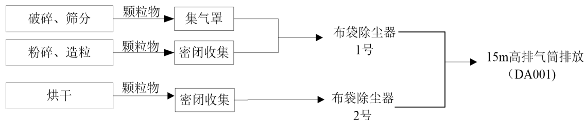
图 4-1 废气收集处理流程
