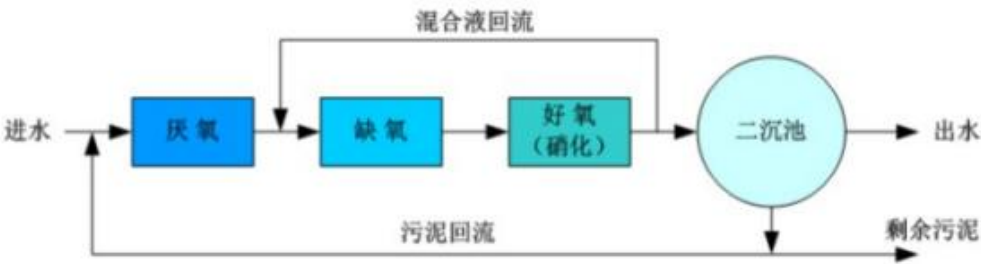
图 4-3 污水处理厂处理工艺流程示意图
