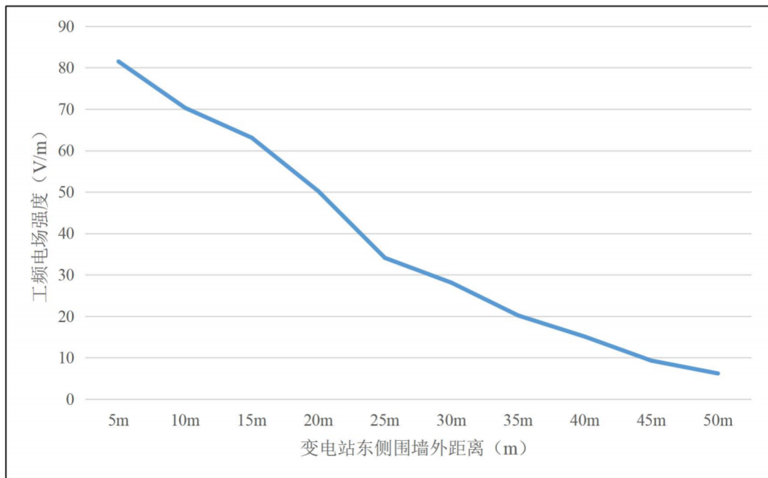
图 3-1 类比变电站断面测点处工频电场强度趋势图
