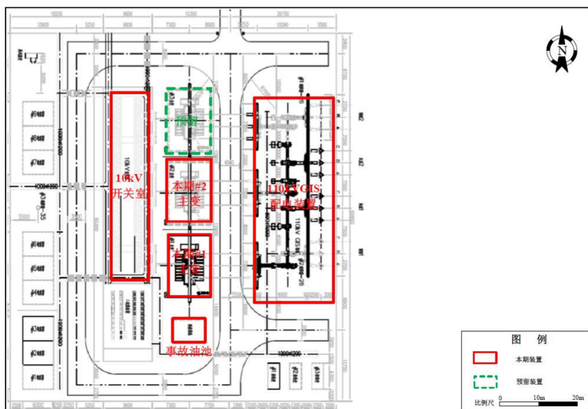
图 3-2 类比变电站总平面布置
