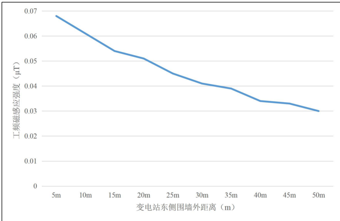
图 3-2 类比变电站断面测点处工频磁感应强度趋势图
