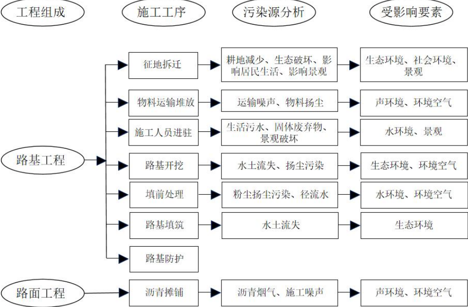
图 4-1 施工工艺及产污节点图
