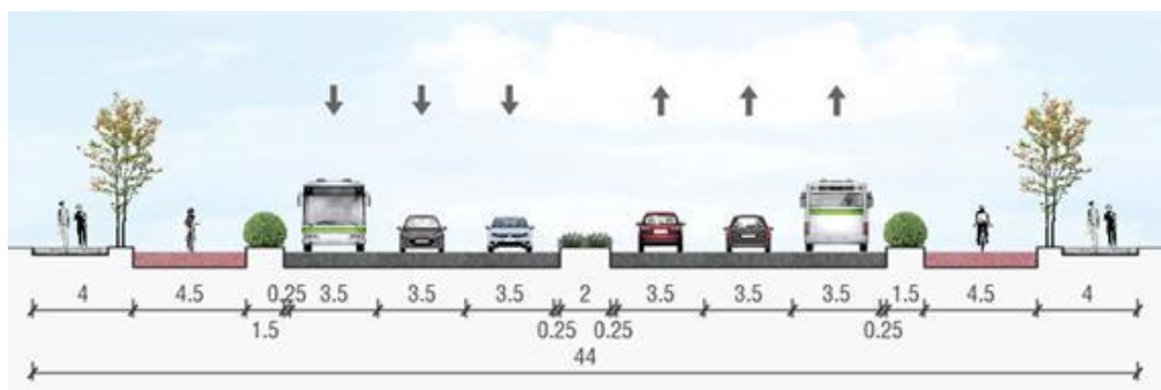
图 2.1-1 站前路一般段横断面图
