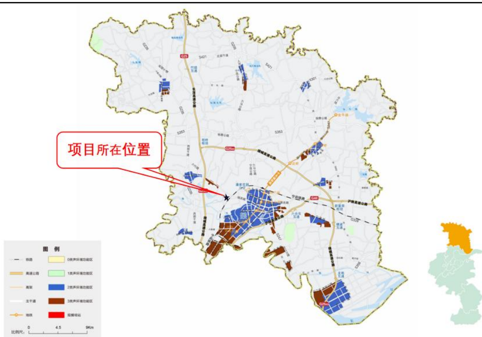
图 3-3 本项目与六合区声环境功能区关系图
