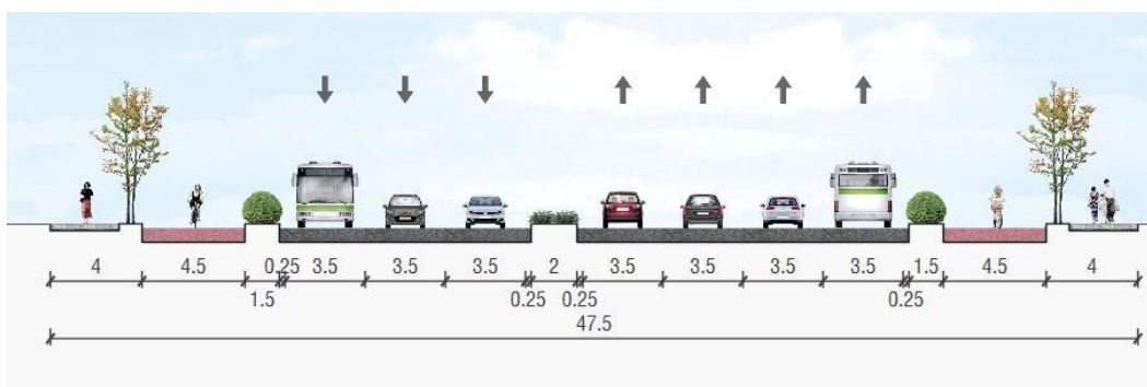
图 2-3 站前路渠化段横断面图
