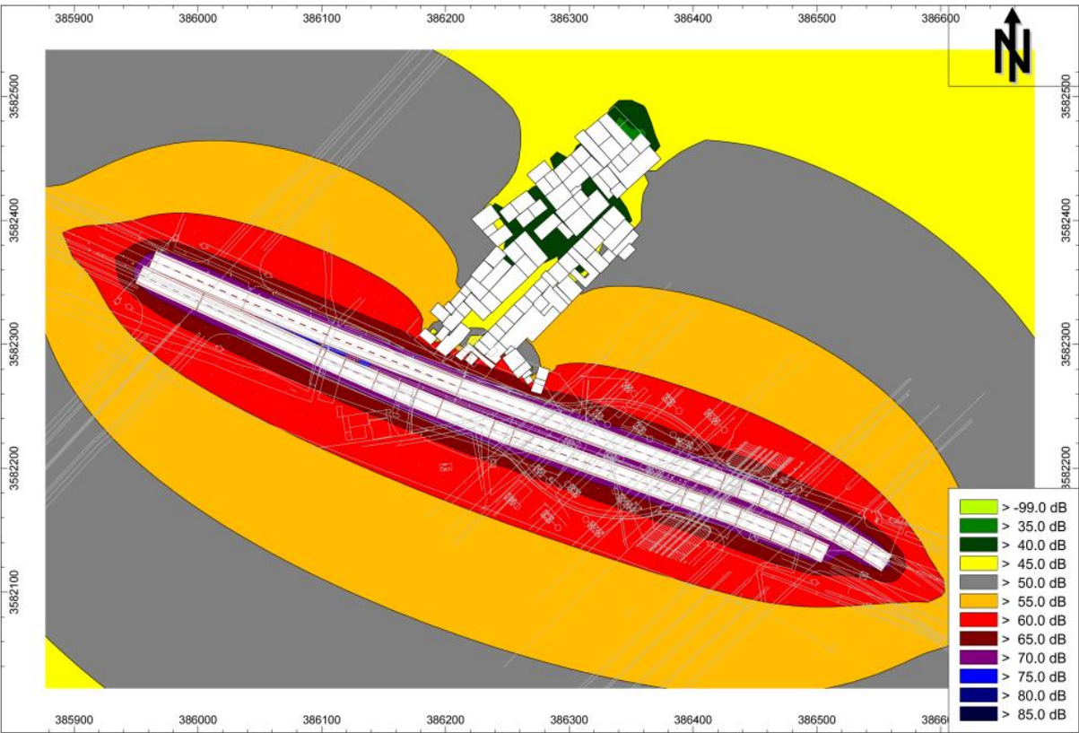
图 5.2-8 昼间等声级线图（中期）
