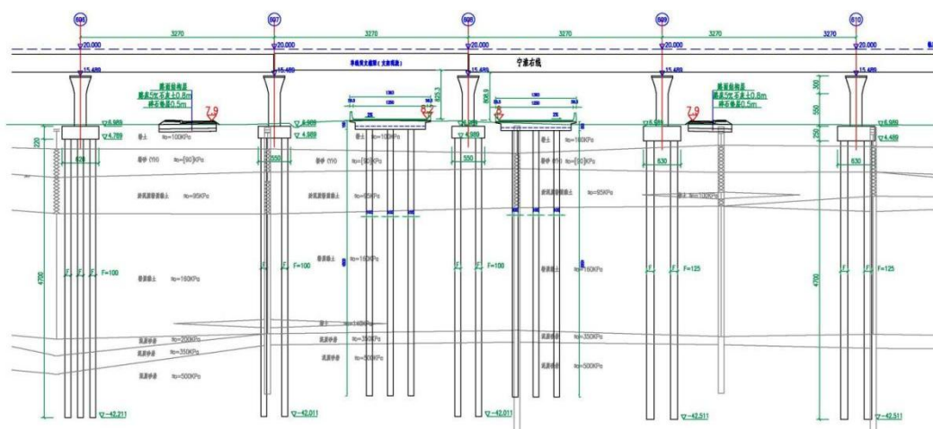
图 2-6 下穿沪渝蓉铁路位置横断面布置图
