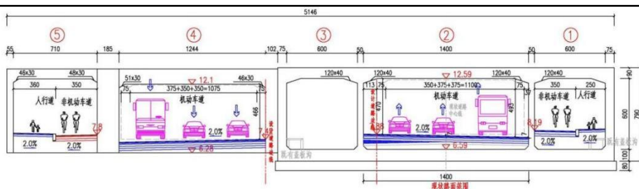
图 2-5 宁启铁路既有框构段横断面布置图
