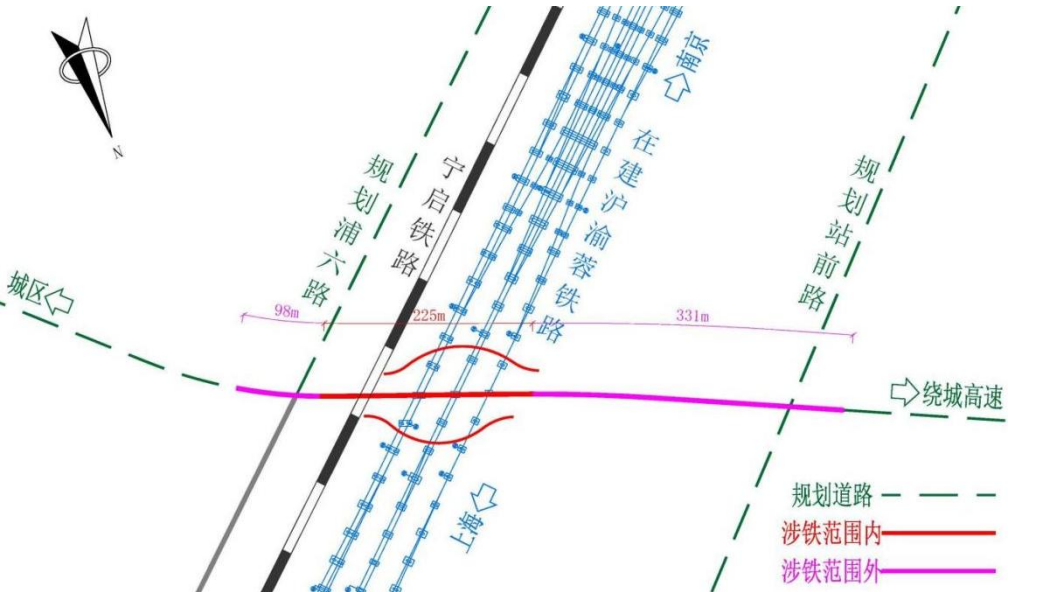
图 2-3 机场大道示意图
