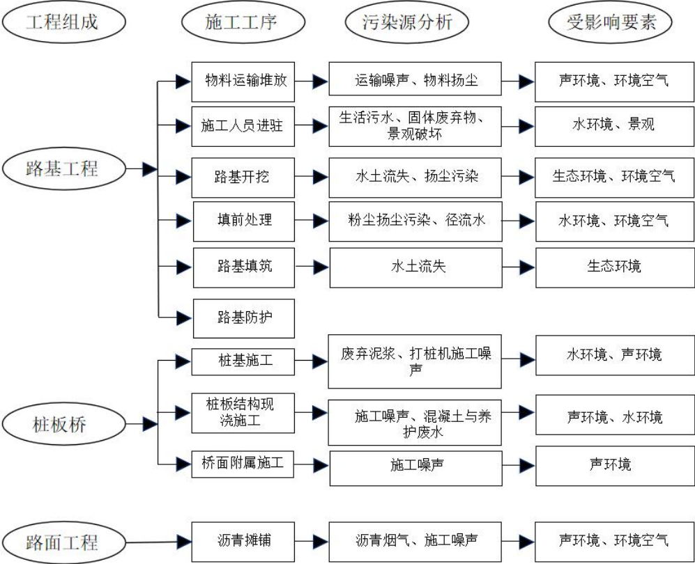
图 4-1 施工工艺及产污节点图
