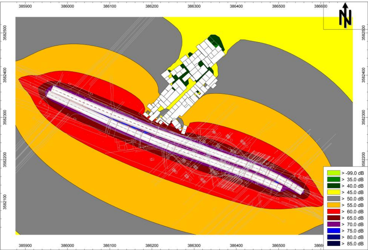
图 5.2-10 昼间等声级线图（远期）
