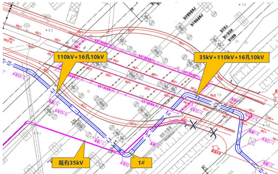
图 2-10 电缆沟平面布置图
