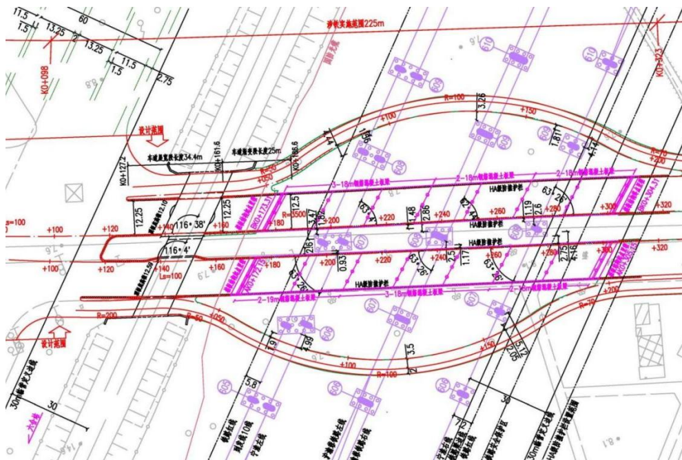
图 2-14 涉铁节点平面布置图
