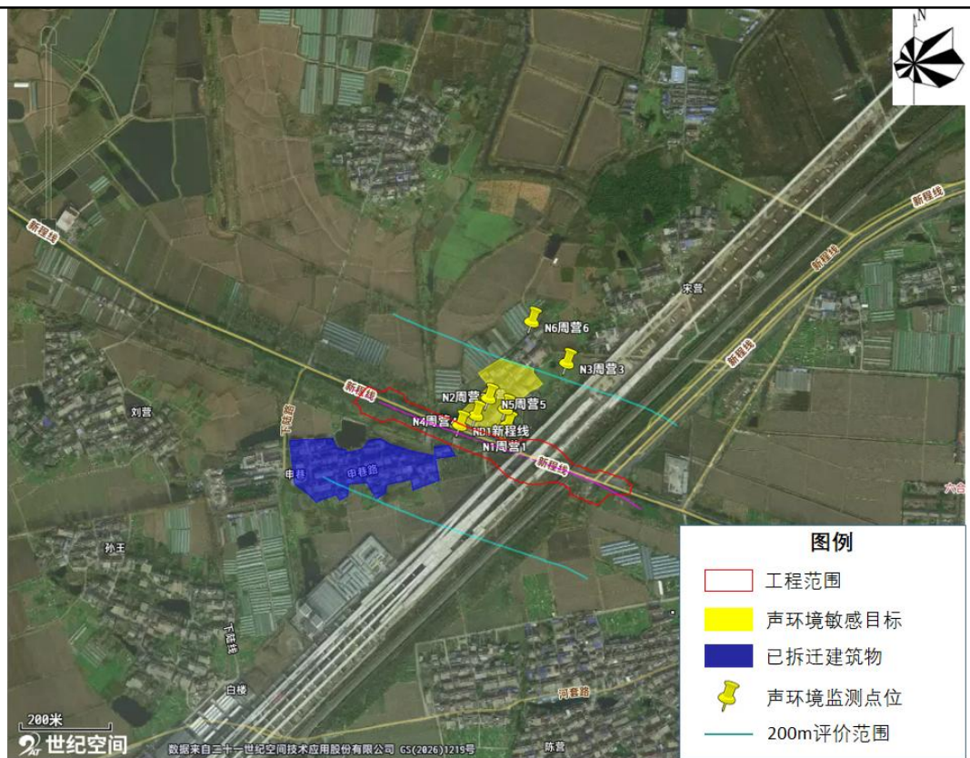
图 2-11 现状已完成市政拆迁范围图
