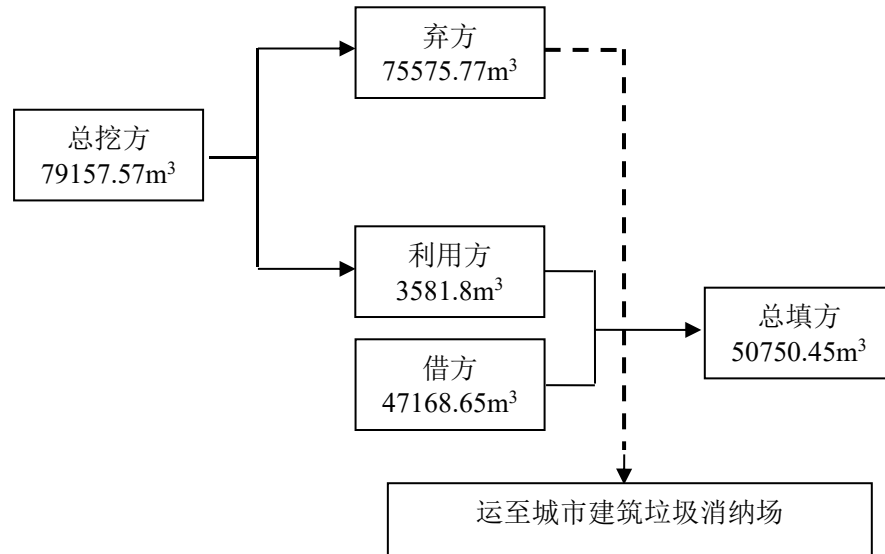
图 2-12 拟建项目路基工程土石方平衡图
