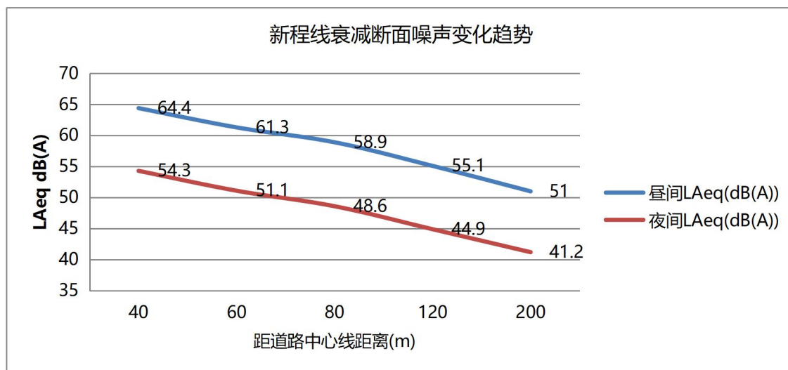
图 4.2-2 衰减监测噪声结果随道路中心线距离变化趋势图
