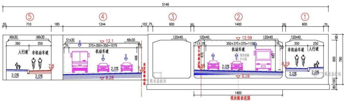
图 2.1-2 宁启铁路既有框构段横断面布置图
