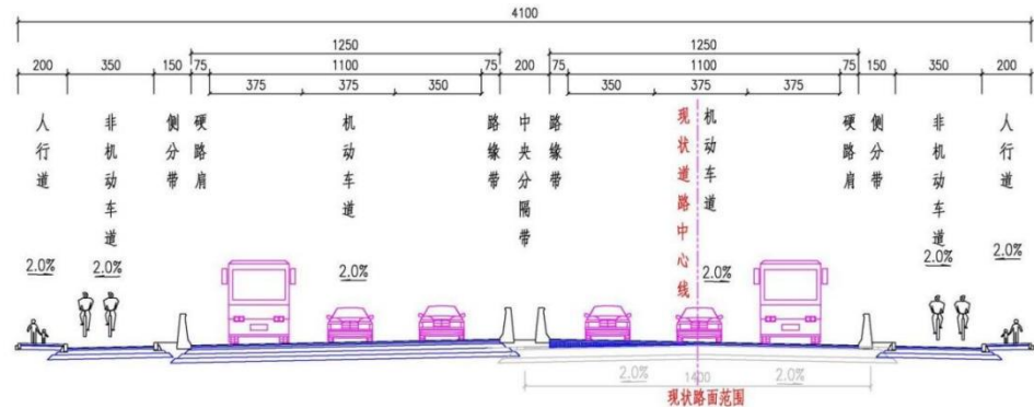
图 2.1-1 一般段路基标准横断面图
