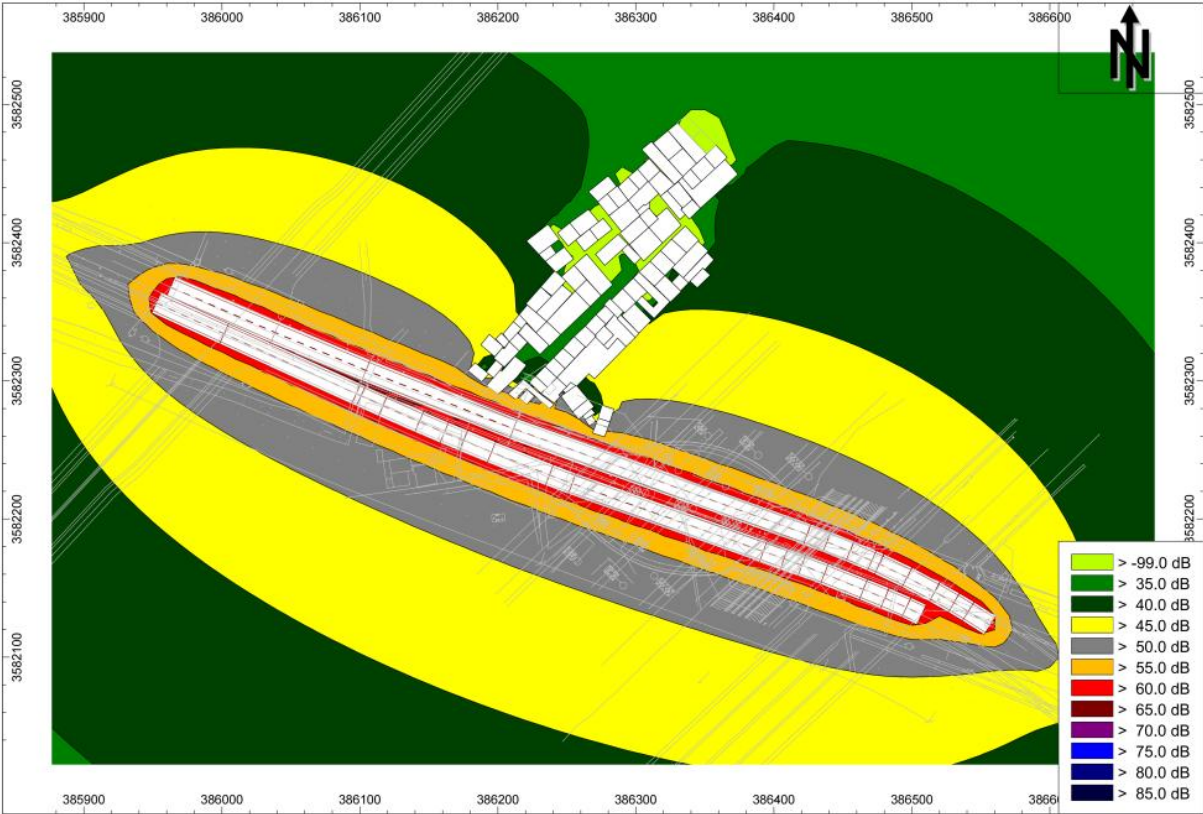
图 5.2-7 夜间等声级线图（近期）
