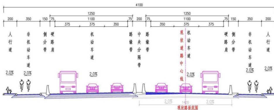
图 2-4 一般段路基标准横断面图
