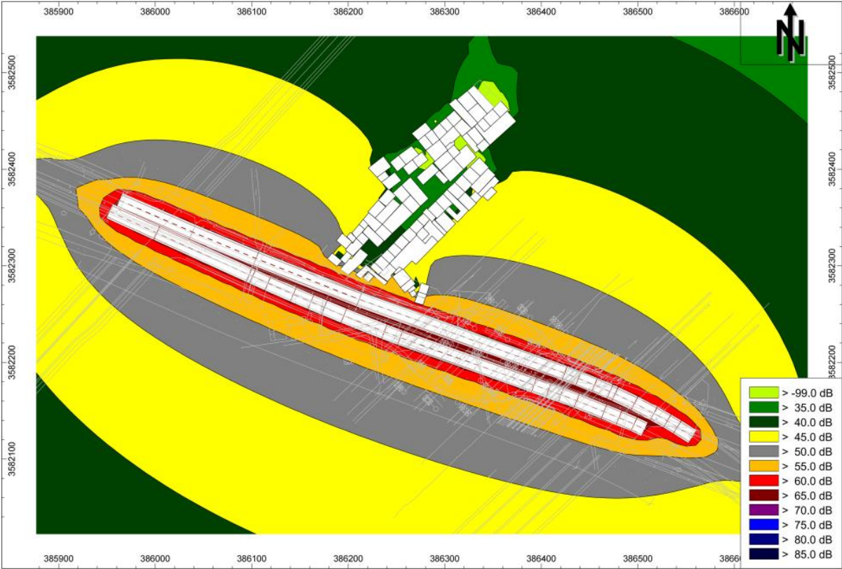
图 5.2-11 夜间等声级线图（远期）
