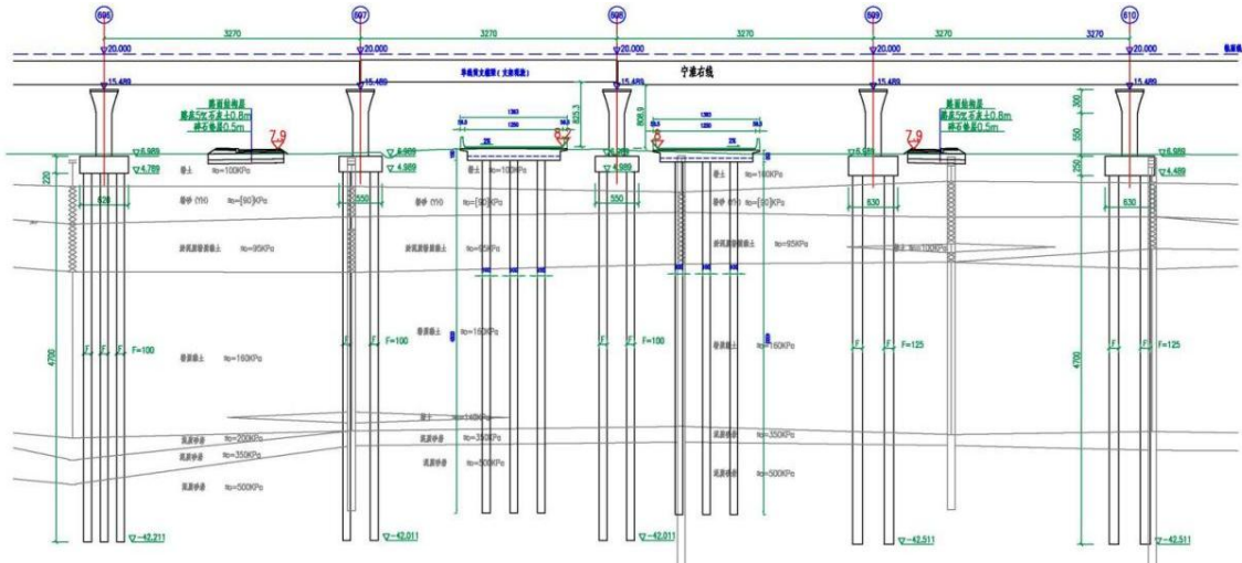
图 2.1-3 下穿沪渝蓉铁路位置横断面布置图
