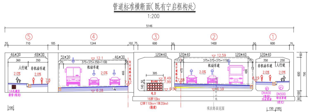
图 2-7 管道标准横断面（既有宁启框构处）
