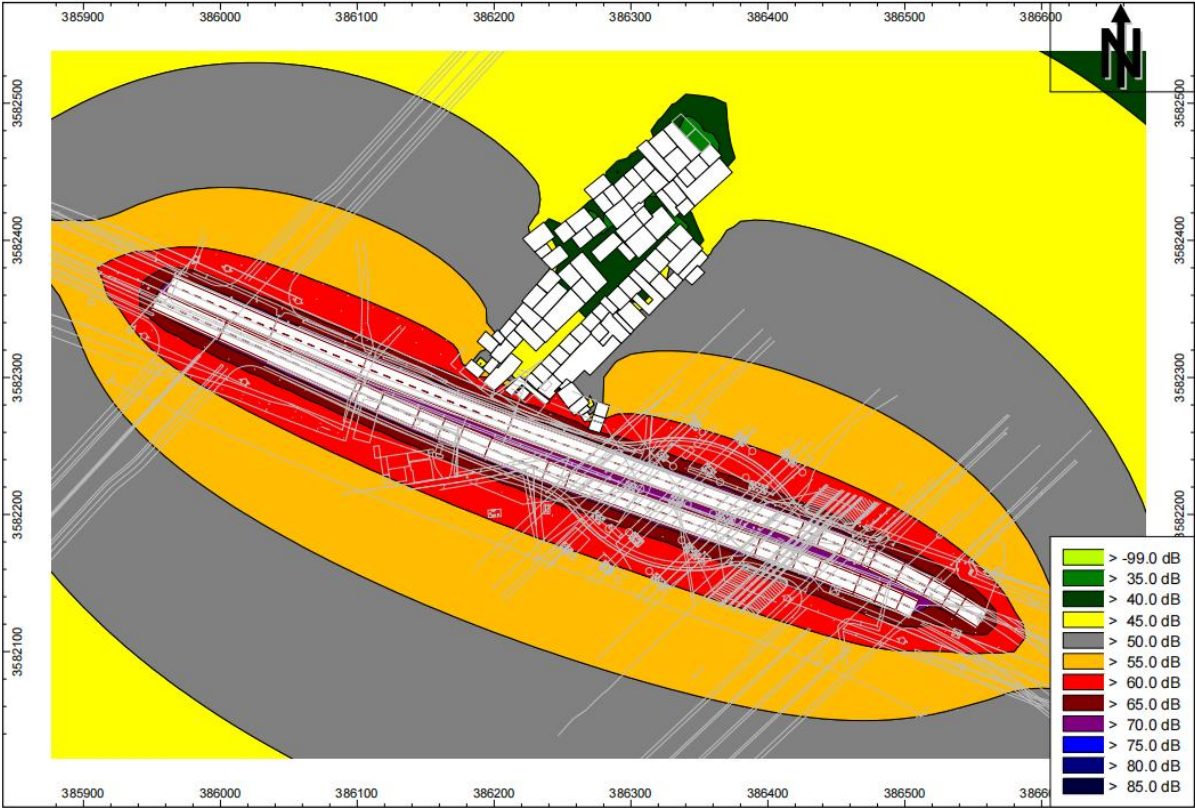
图 5.2-6 昼间等声级线图（近期）
